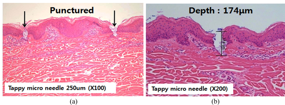
그림 7. 마이크로니들이 침투된 돼지피부 절편의 광학현미경 이미지
