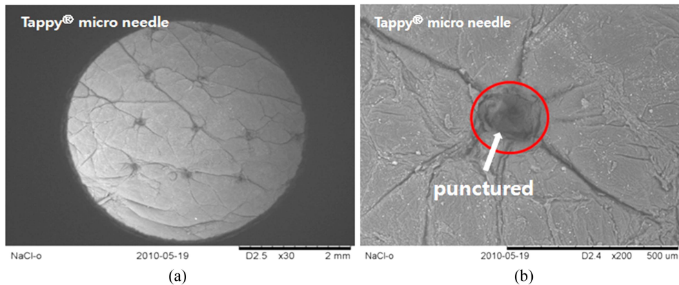
그림 6. 마이크로니들 적용 후 돼지피부 표면 SEM 이미지
