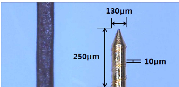
그림 3. 마이크로니들과 머리카락 두께 비교 사진 Fig. 3. Picture of hair and micro needle to compare to thickness (left : Hair, Right : Micro needle of Tappy®)
