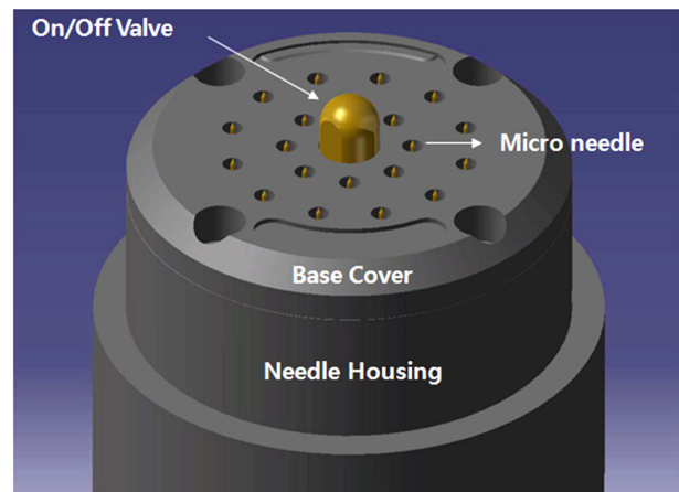
그림 2. 마이크로니들 장치 모식도
